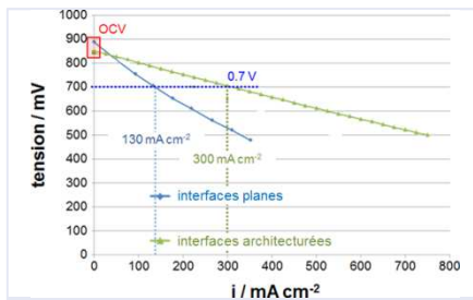
Courbes i/v de piles de type SOFC à interfaces planes et architecturées
