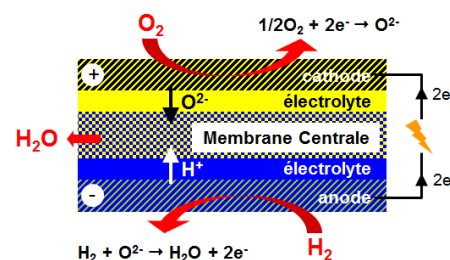
Développement des technologies SOFC de rupture. Cellule à trois chambres.
